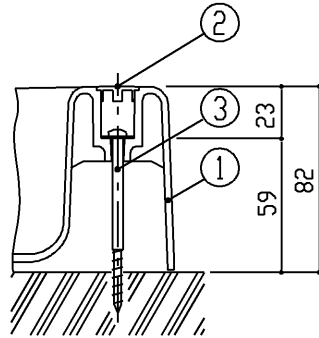
固定部詳細(1/3)
